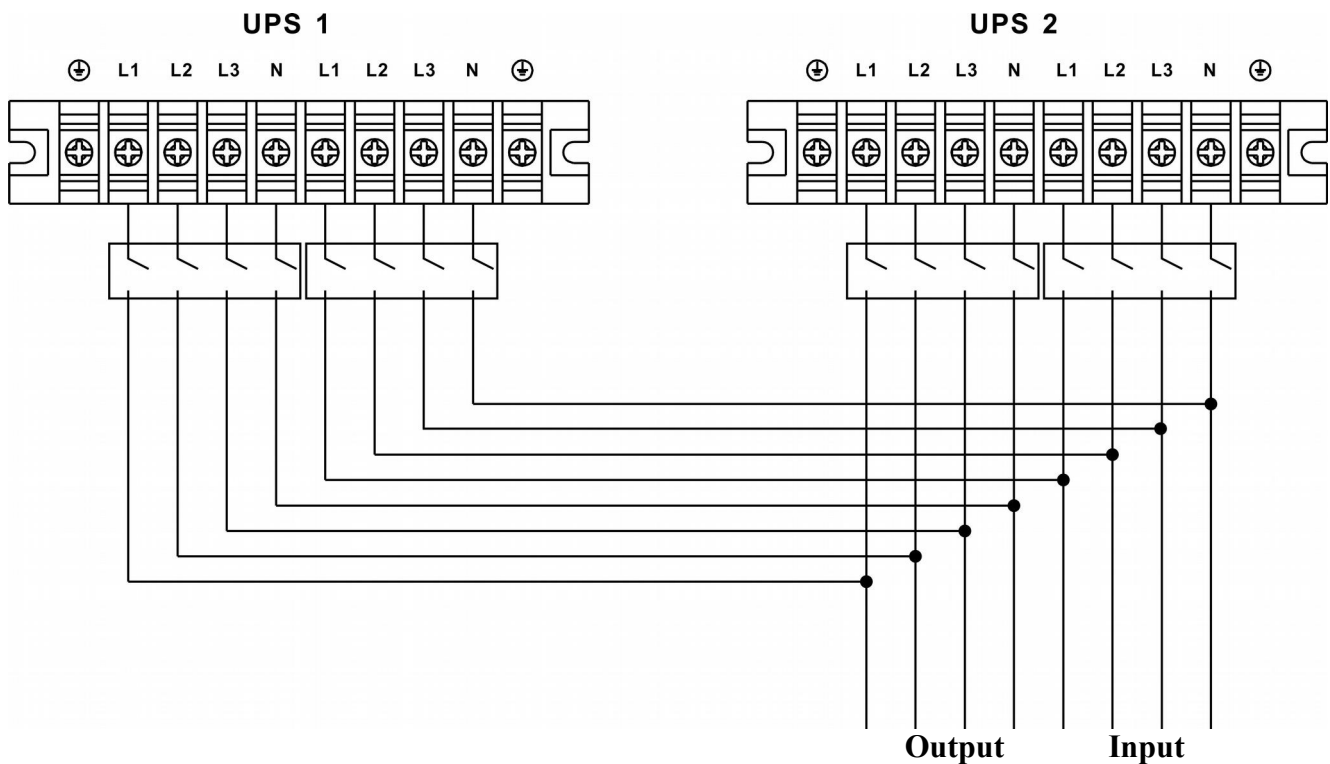
Рис.2-4-2 Подключение в параллельную систему ИБП XE 10WB/ 20WB (на примере двух ИБП).
