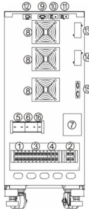
ИБП 10 кВА модель (S)
