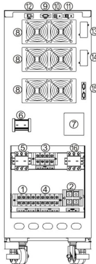
ИБП 15 кВА - 30 кВА модель(S)
