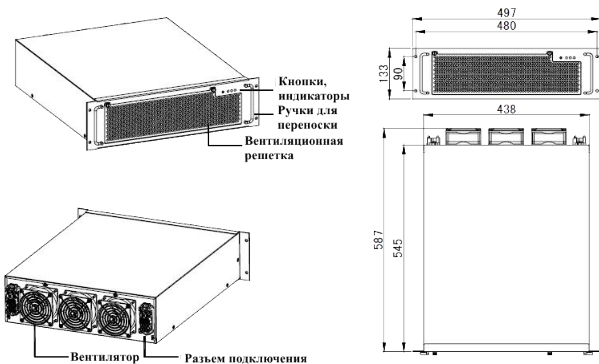
Рис.3-2 Внешний вид и габаритные размеры силового модуля
