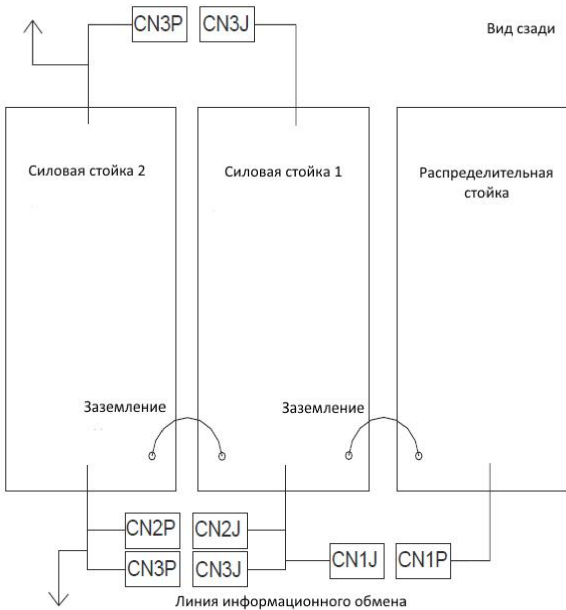
Рис.4-12 Схема объединения распределительной и силовых стоек для Monolith XM260, XM520
